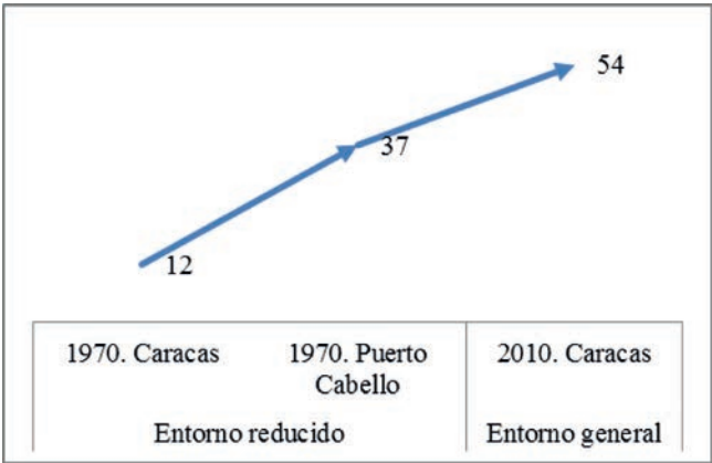
Gráfico 2. Comparación temporal de la variante elidida [Ø] en el español venezolano (%)
